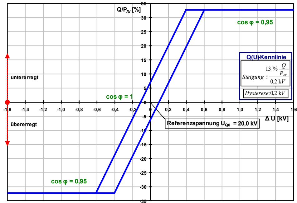
Abb. 53: Q(U) -Kennlinien-Regelung (ehemals Bild L.1)
