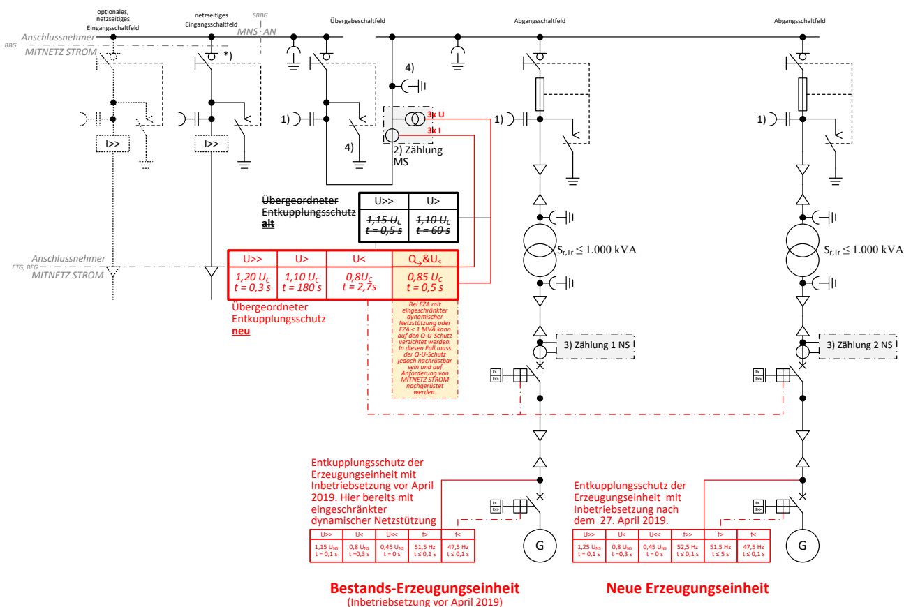
Abb. 29: (ehemals D4b): \leq 20 -kV-Anbindung von zwei Erzeugungseinheiten (Bestands-Erzeugungseinheit; neue Erzeugungseinheit)
