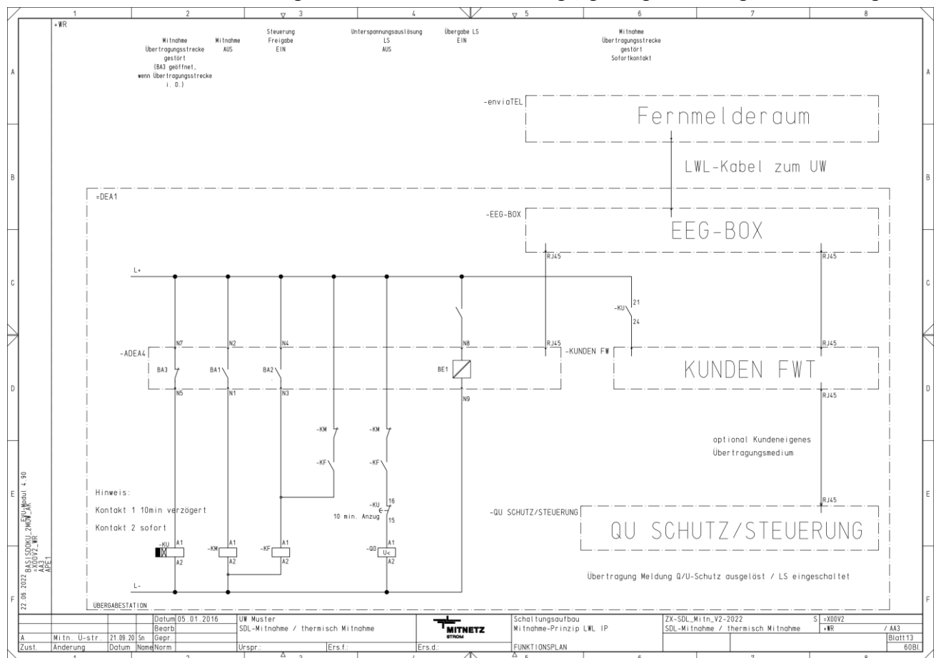
Abb. 51: Schaltungsaufbau der LWL-Kabelverbindung zwischen der Übergabestation und dem MITNETZ STROM-Umspannwerk (Standardfall)
