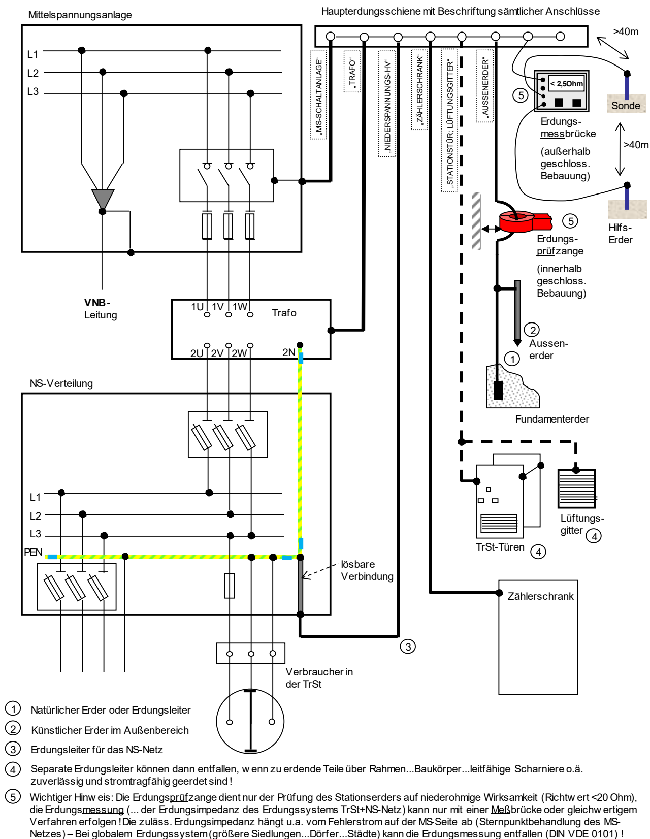
Abb. 8: Gemeinsame Mittel- und Niederspannungs-Erdungsanlage in einer Übergabestation
