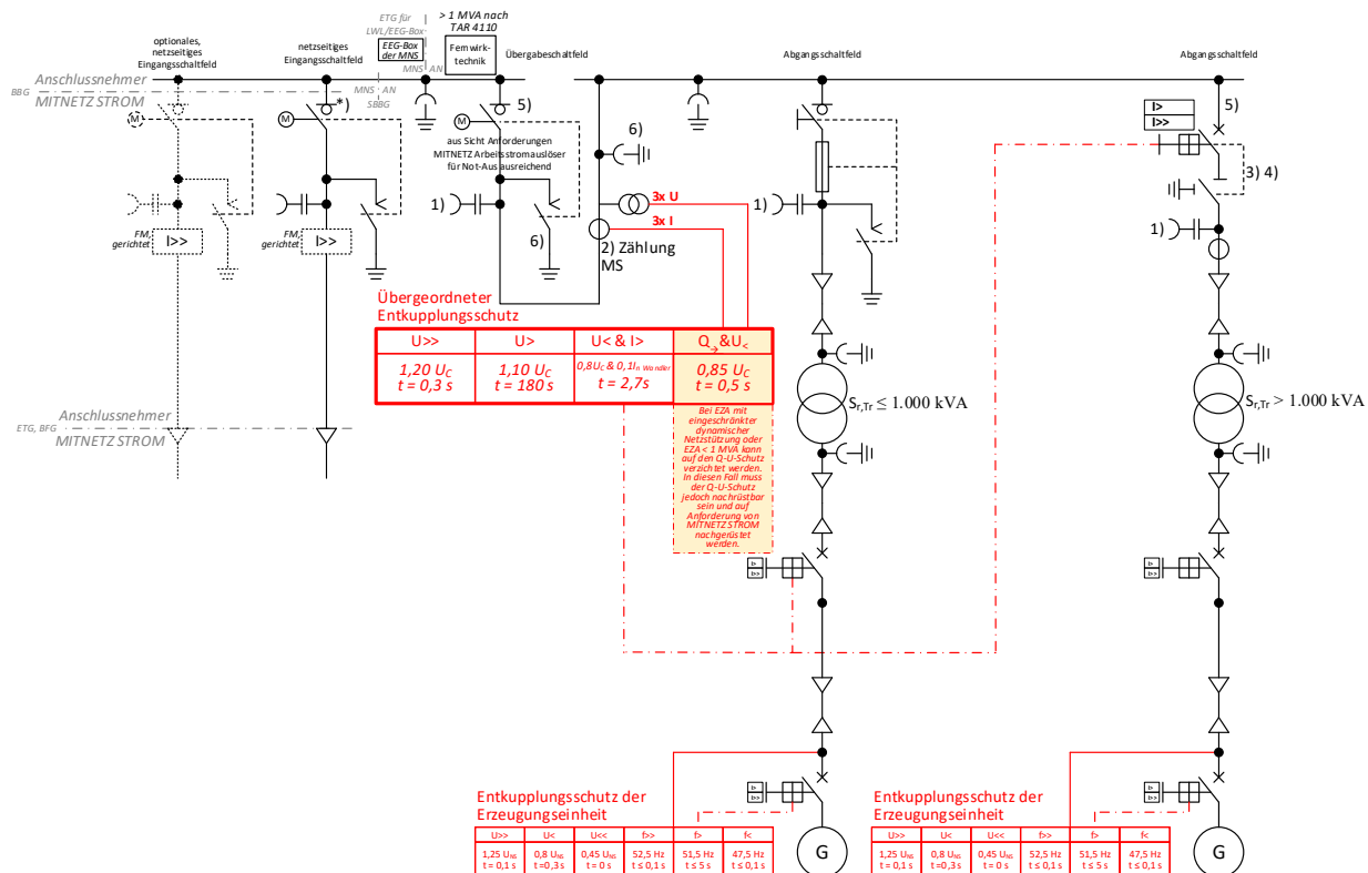
Abb. 28: (ehemals D4a): \leq 20 -kV-Anbindung von zwei Erzeugungseinheiten ( 1x > 1MVA , 1x \leq 1MVA ) über jeweils einen Transformator
