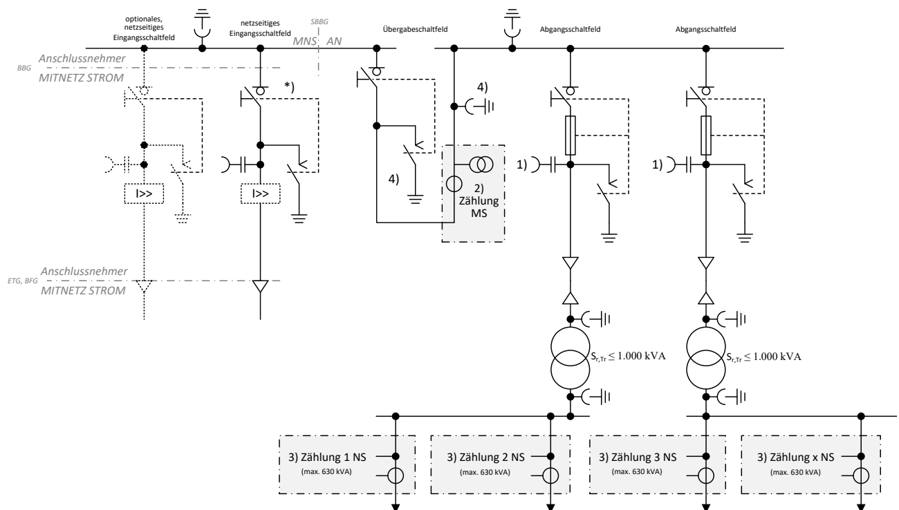
Abb. 25: (ehemals D2a): ≤ 20-kV-Anbindung mit zwei Abgangsfeldern; Transformatoren ≤ 1 MVA mit Übergabe-Lasttrennschalter
