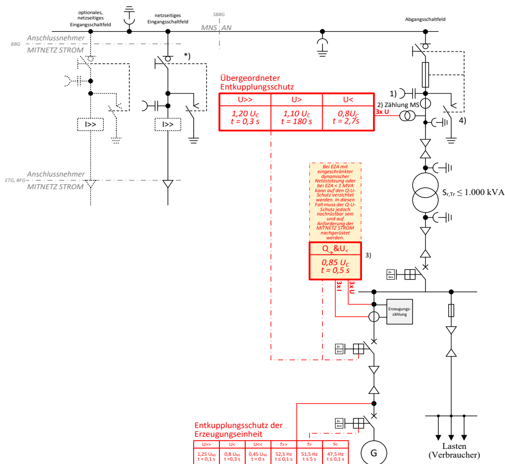
Abb. 33: (ehemals D5a): \leq 20 -kV-Anbindung einer Mischanlage über einen Transformator
