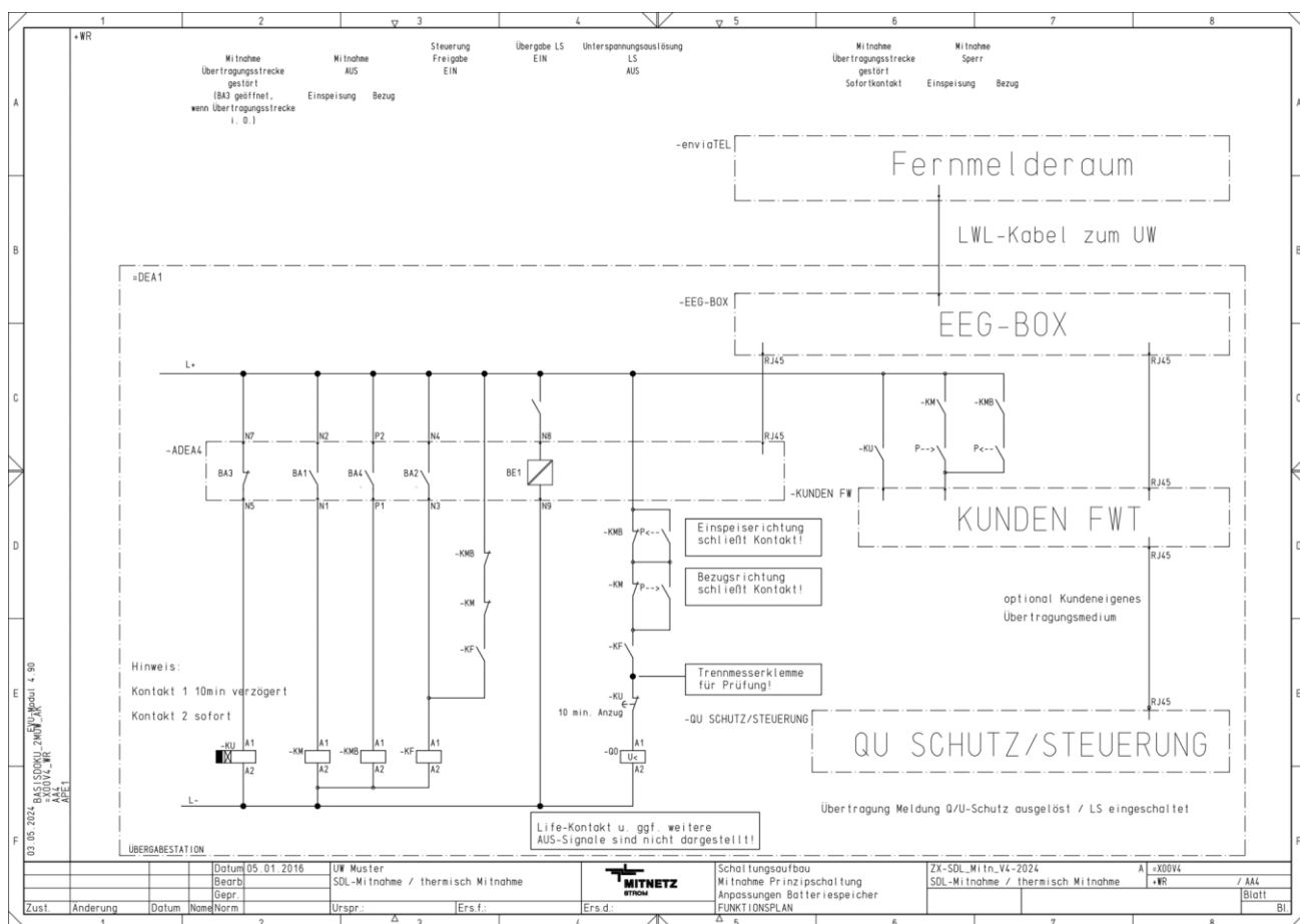
Abb. 52: Schaltungsaufbau der LWL-Kabelverbindung zwischen der Übergabestation und dem MITNETZ STROM-Umspannwerk (richtungsabhängig)
