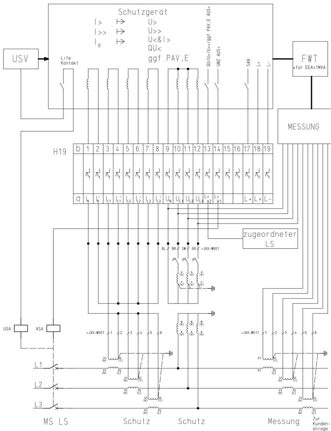
Abb. 46: Wandlerverdrahtung Anbindung UMZ / übergeordneter Entkopplungsschutz
