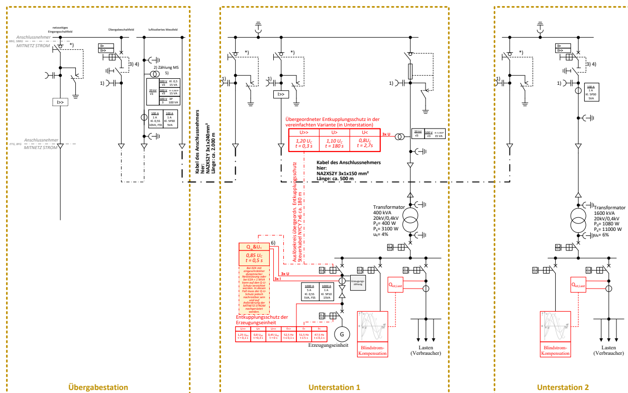
Abb. 37: (ehemals D5e): ≤ 20-kV-Anbindung von zwei Unterstationen mit Blindstromkompensation der Lasten der Bezugsanlage und vereinfachter Variante des übergeordneten Entkopplungsschutz
