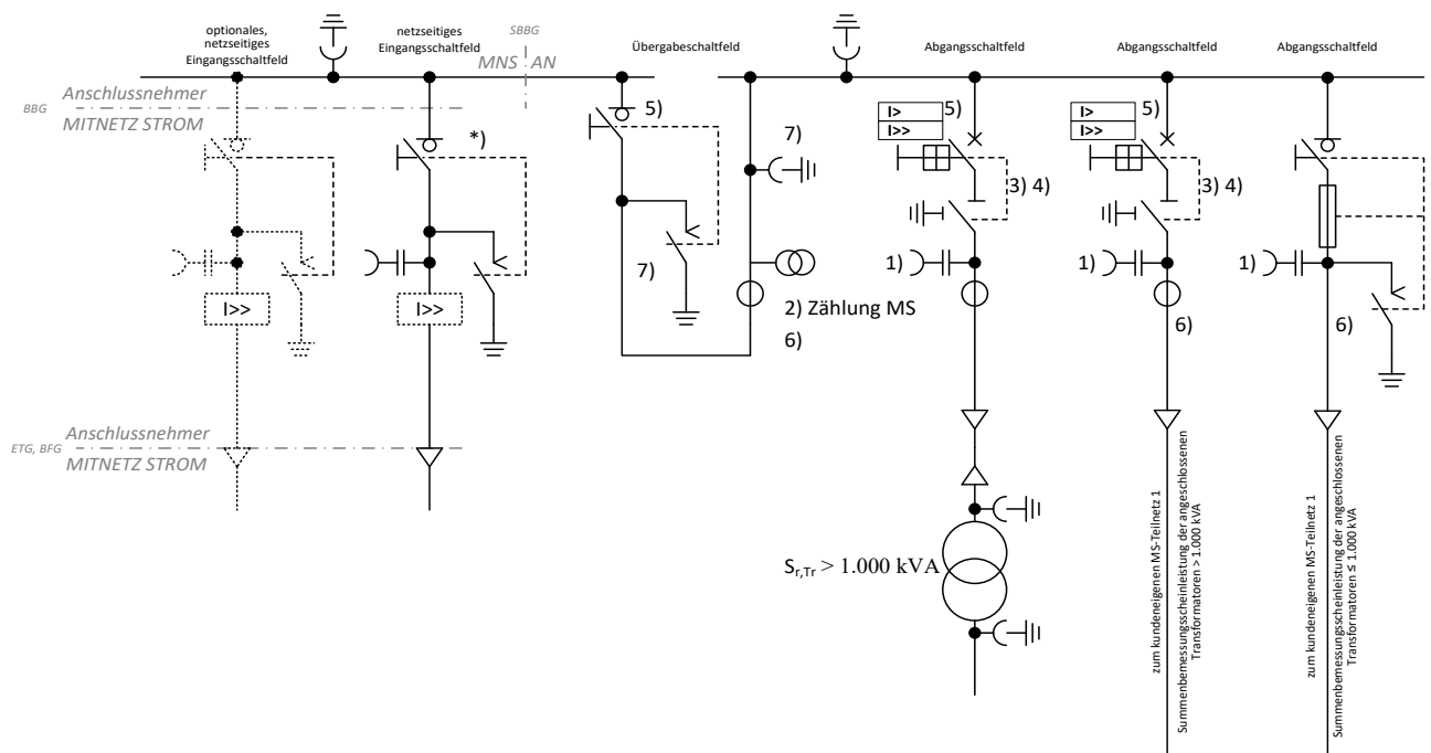
Abb. 26: (ehemals D2b): ≤ 20-kV-Anbindung mit drei Abgangsfeldern (ein Transformator > 1 MVA, zwei Kabelabgangsfelder [kundeneigenes MS-Netz und ein Transformator ≤ 1 MVA bzw. ein Transformator > 1 MVA] mit Übergabe-Lasttrennschalter
