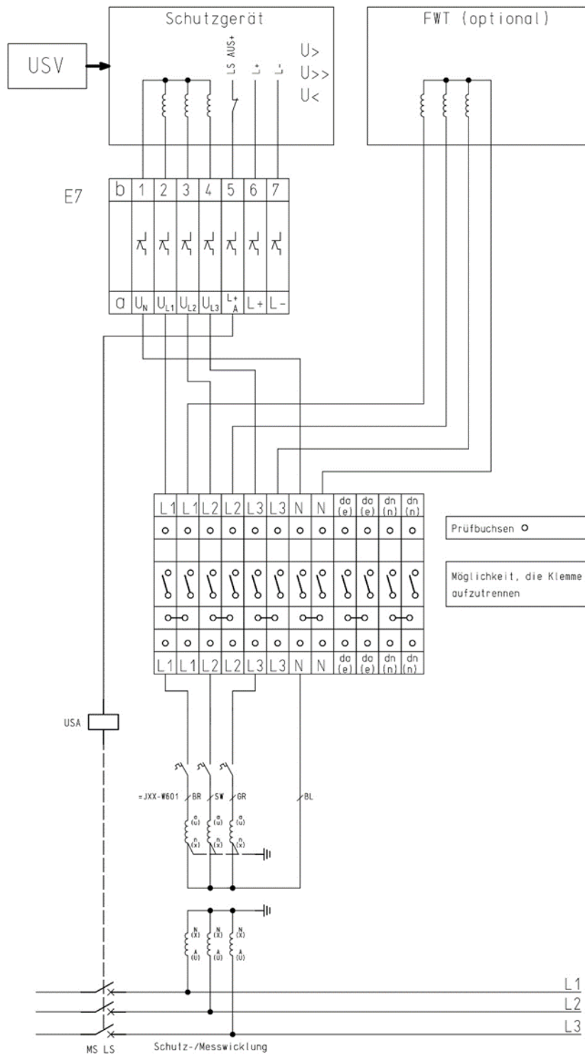
Abb. 48: Wandlerverdrahtung Anbindung übergeordneter Entkupplungsschutz / Fernwirkgerät
