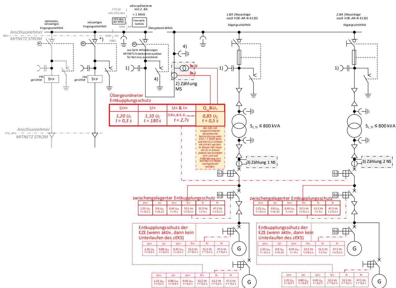
Abb. 32: (ehemals D4e): ≤ 20-kV-Anbindung von zwei Bauabschnitten einer PV-Anlage mit je 750 kVA (spätestens ab 2.BA mit FWT, in diesem Fall im 1.BA mit FRE)
