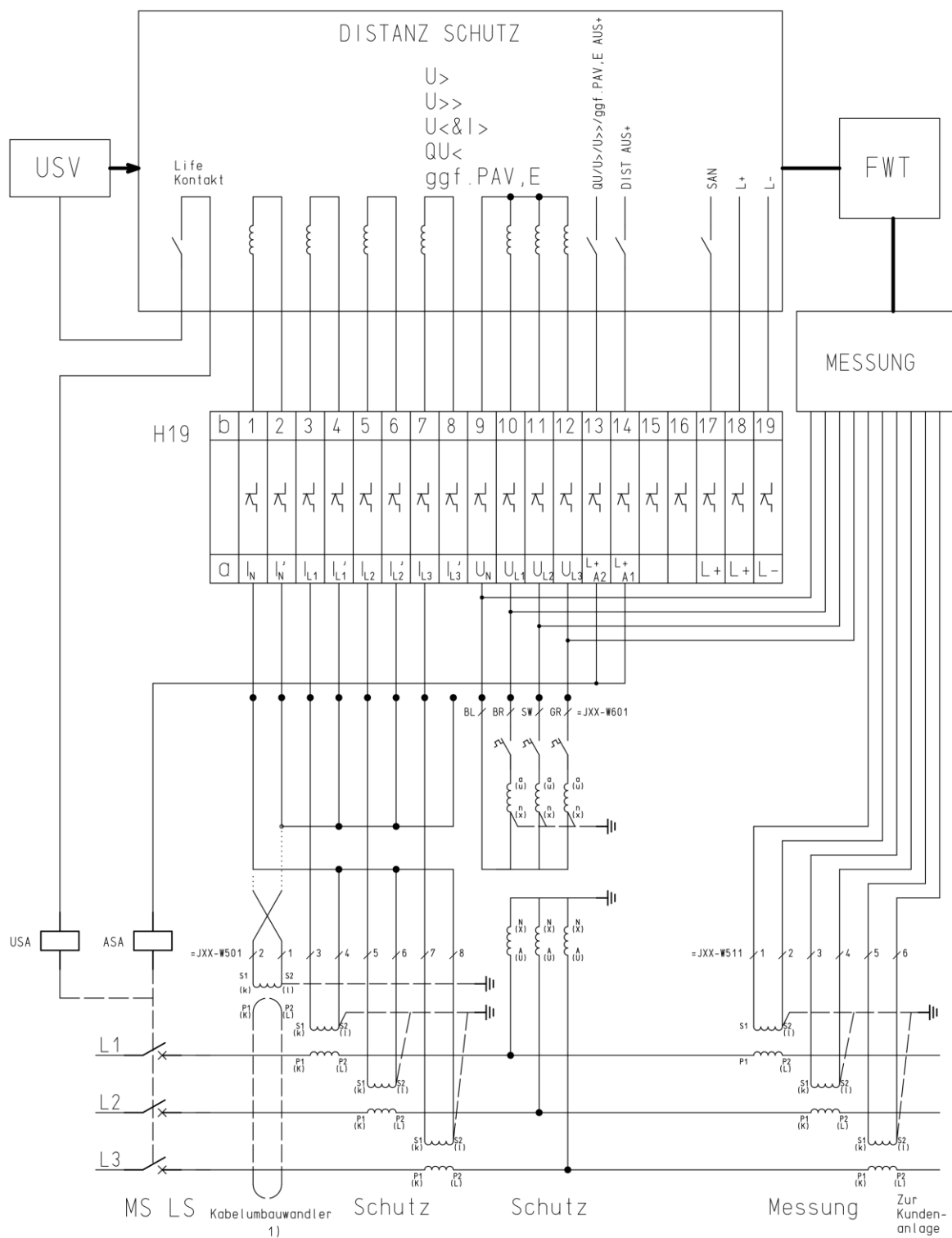
Abb. 50: Wandlerverdrahtung Anbindung Distanzschutz
