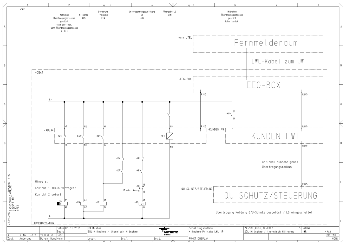
Abb. 51: Schaltungsplan der LWL-Kabelverbindung zwischen der Übergabestation und dem MITNETZ STROM-Umspannwerk (Standardfall)
