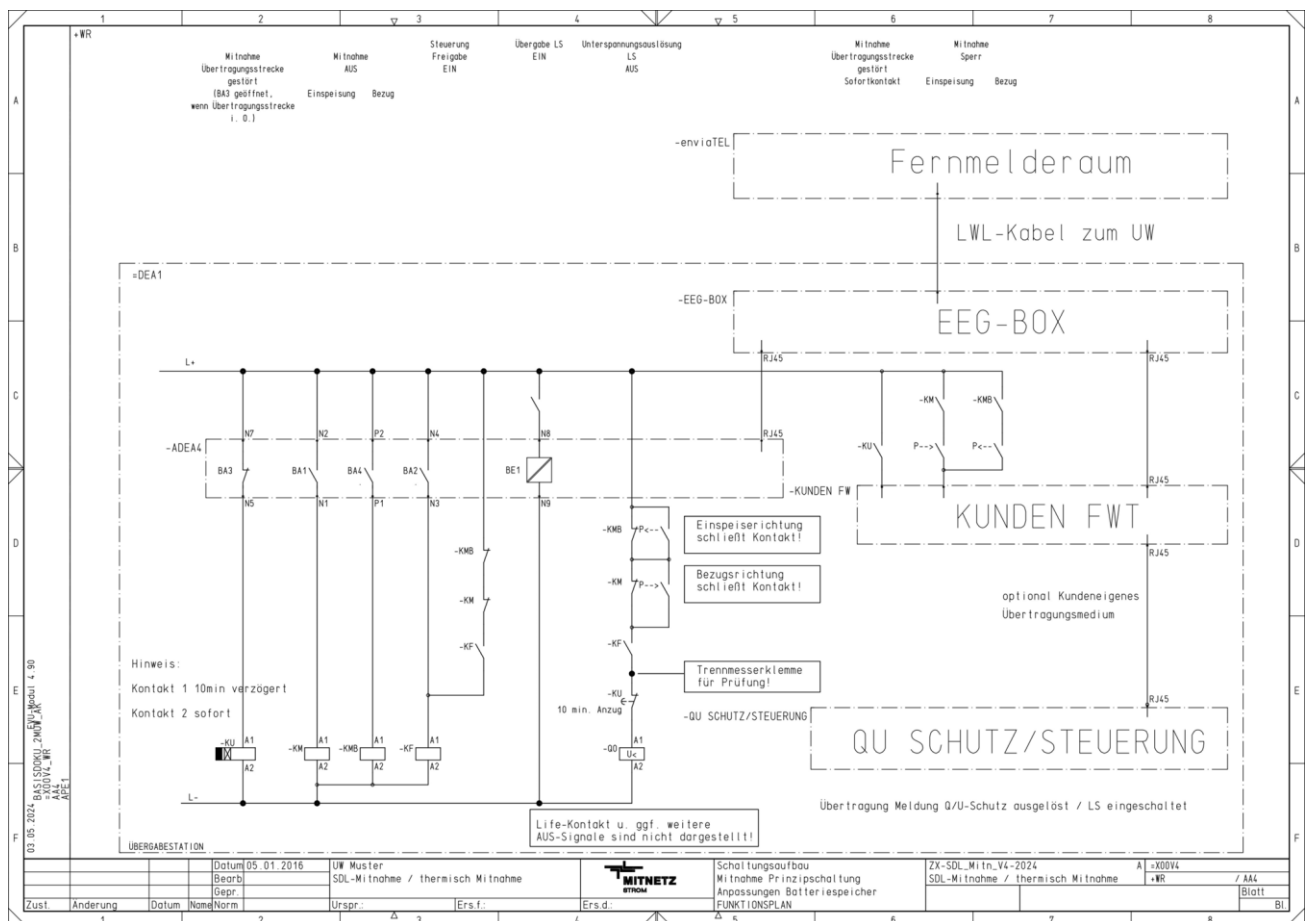
Abb. 52: Schaltungsaufbau der LWL-Kabelverbindung zwischen der Übergabestation und dem VN Plauen-Umspannwerk (richtungsabhängig)
