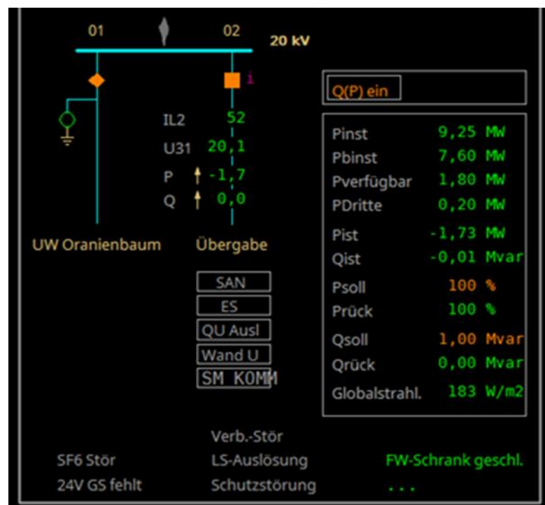
Abb. 22: Beispiel der Darstellung eines MS-Sammelschienen-Anschlusses in einem Umspannwerk im Netzleitsystem der VN Plauen (Die Darstellung eines MS-Netz-Anschlusses erfolgt bis auf Q_{\text{soll}}/Q_{\text{rück}} in gleichem Umfang.)
