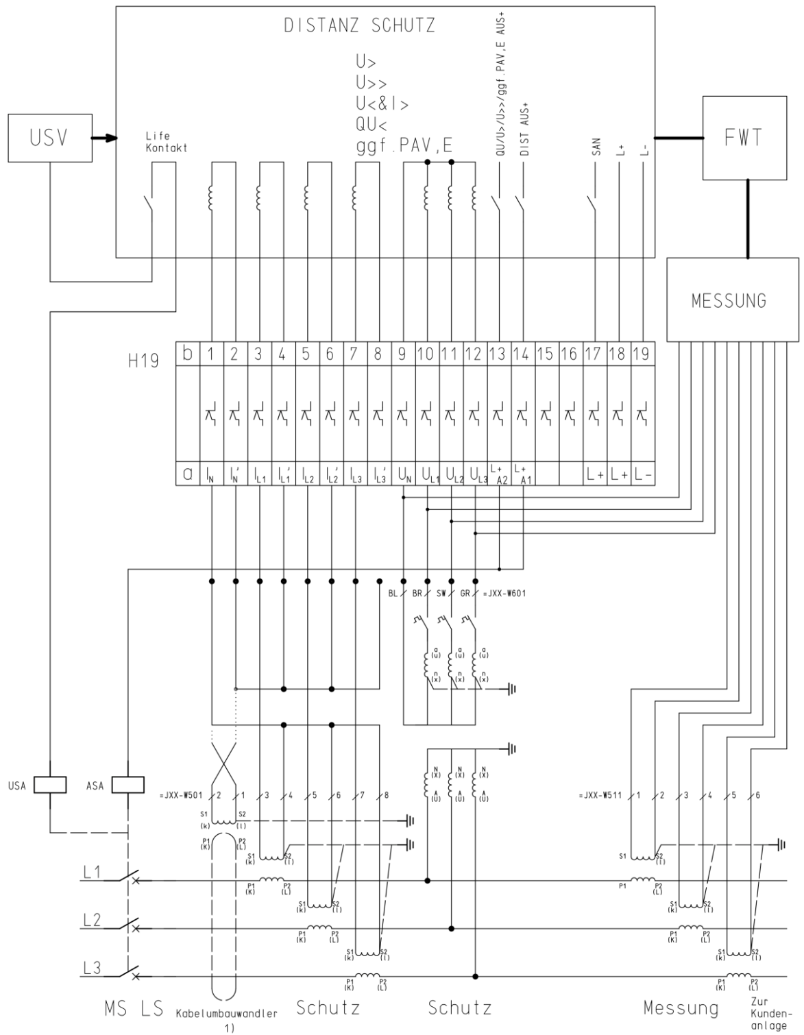
Abb. 50: Wandlerverdrahtung Anbindung Distanzschutz
