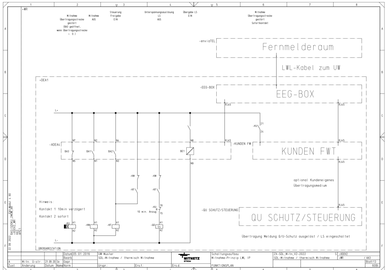
Abb. 51: Schaltungsaufbau der LWL-Kabelverbindung zwischen der Übergabestation und dem VN Plauen-Umspannwerk (Standardfall)
